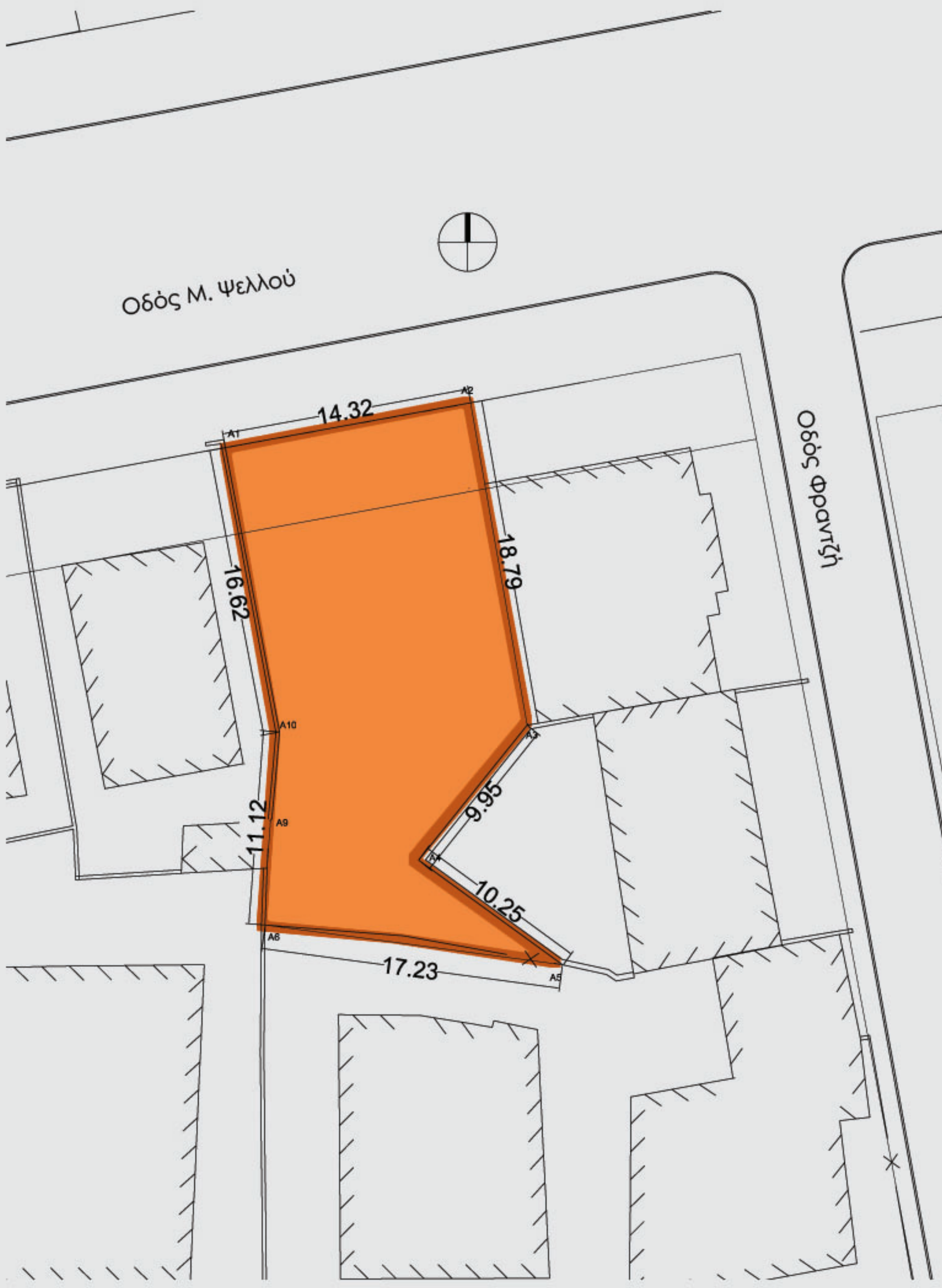
Τοπογραφικό διάγραμμα οικοπέδου στην οδό Μ.Ψελλού 26 Ε= 395 τ.μ
